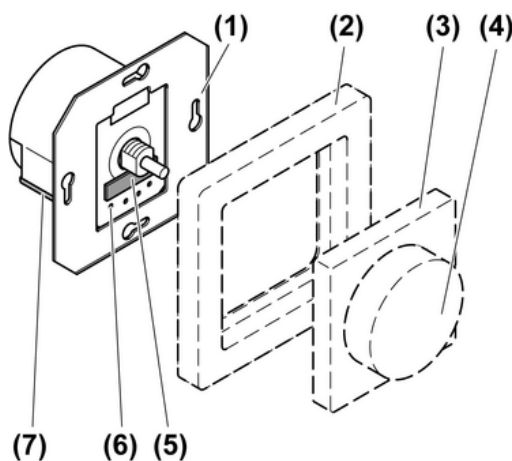
Рис.1: конструкция прибора
